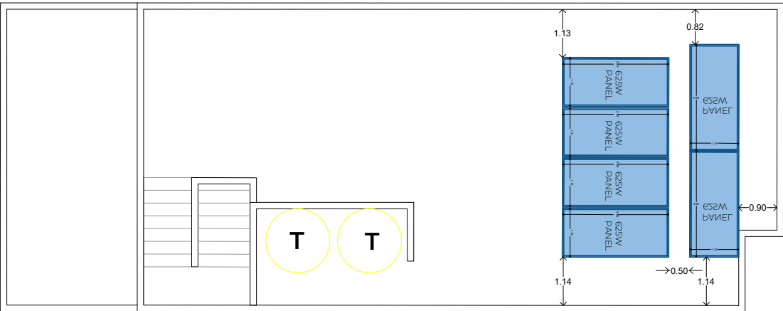
PLANTA PANELES
