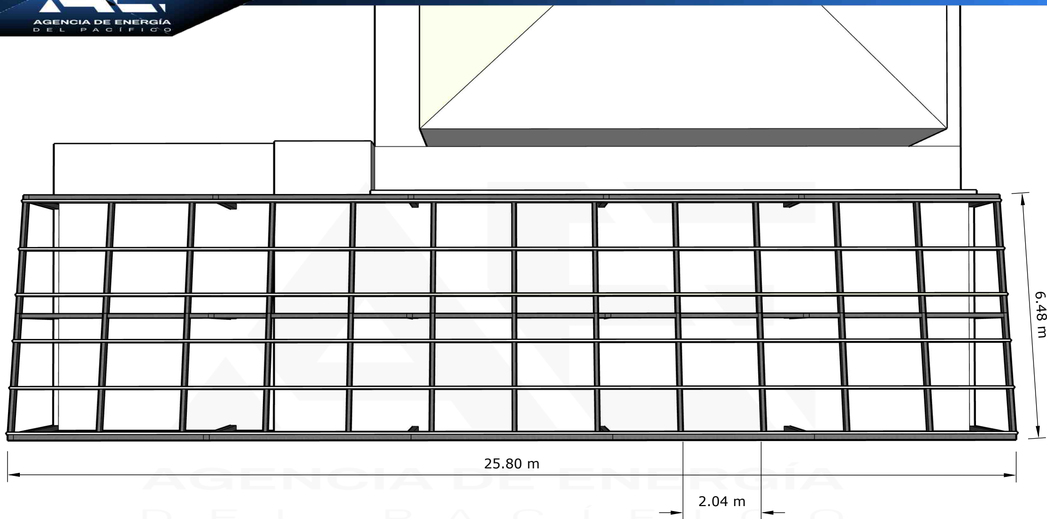
Estructura metálica lado norte
